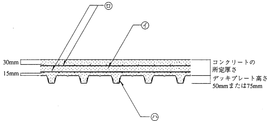
B-B断面図
