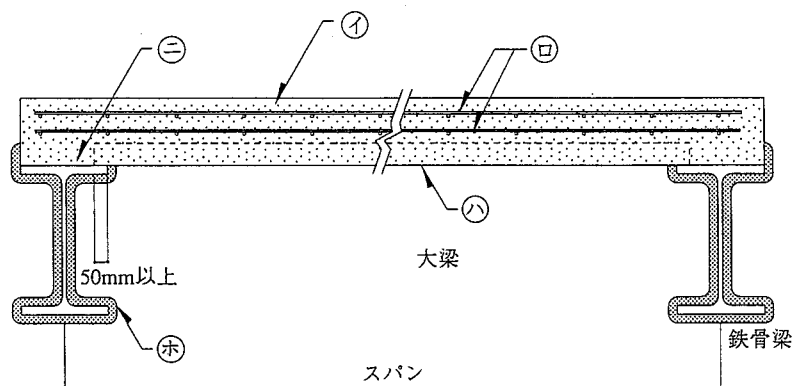
A-A断面図
