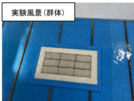
実験水路
